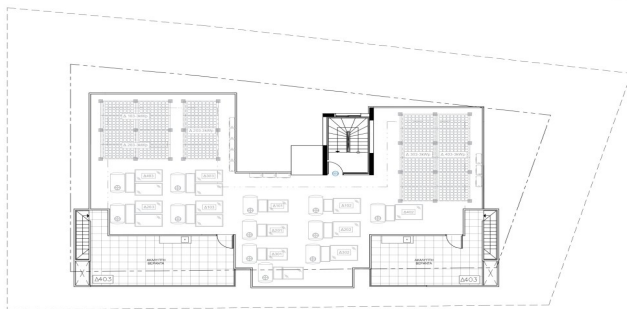
KATONHI 5-OY OPOROY KIMMA 1:500
